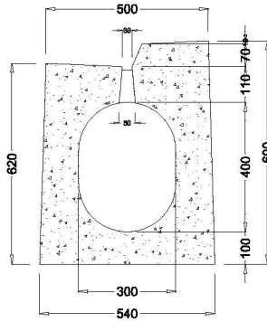
PROFILO RIALZATO mod. eurobeton 30/40 A7 peso 2100 kg. cad.
