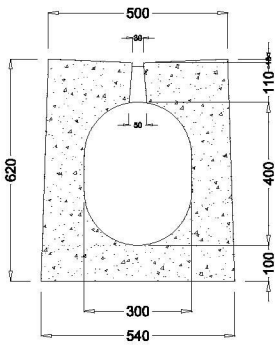
PROFILO PIANO mod. eurobeton 30/40 peso 2000 kg. cad.
