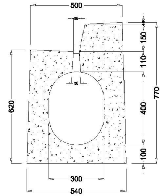
PROFILO RIALZATO mod. eurobeton 30/40 A15 peso 2300 kg. cad.
