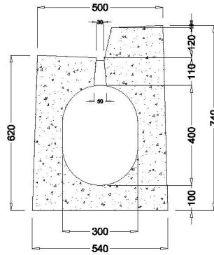
PROFILO RIALZATO mod. eurobeton 30/40 A12 peso 2200 kg. cad.
